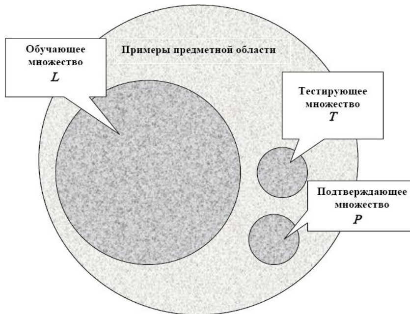
Рисунок 2.2 – Поділ прикладів предметної області на навчальне безліч L , тестуюча безліч T і підтверджує безліч P
