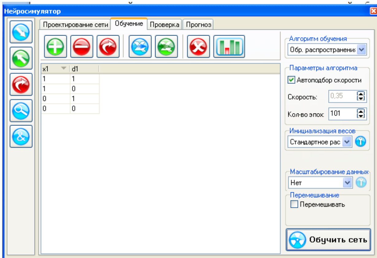
Рисунок 2.4 – Приклад навчання нейронної мережі в програмі Нейросимулятор
