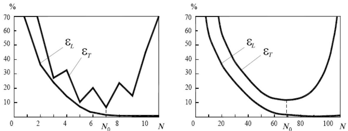
Рисунок 2.6 – Характерні залежності помилки навчання \epsilon_L і помилки Узагальнення (тестування) \epsilon_T від кількості нейронів прихованих шарів перцептрона N
