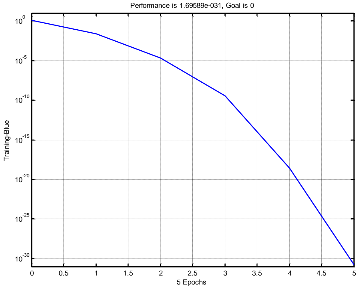
Рисунок 6.2 – Графік навчання двошарового перцептрона
