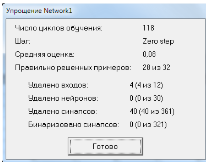
Рисунок 7.5 - Зміна параметрів мережі при її спрощенні
