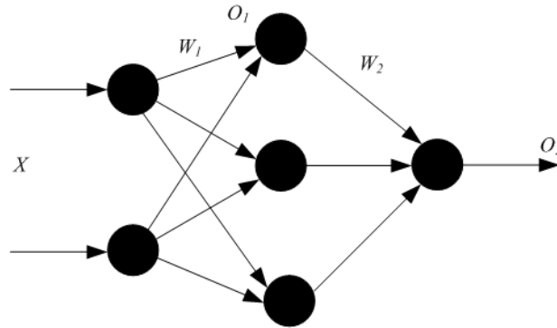
Рисунок 6.1 – Багатошаровий перцептрон
