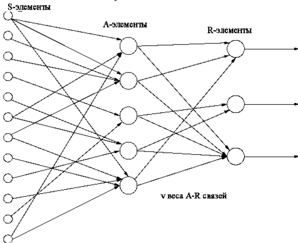
Рисунок 5.1 – Перцептрон Розенблатта
