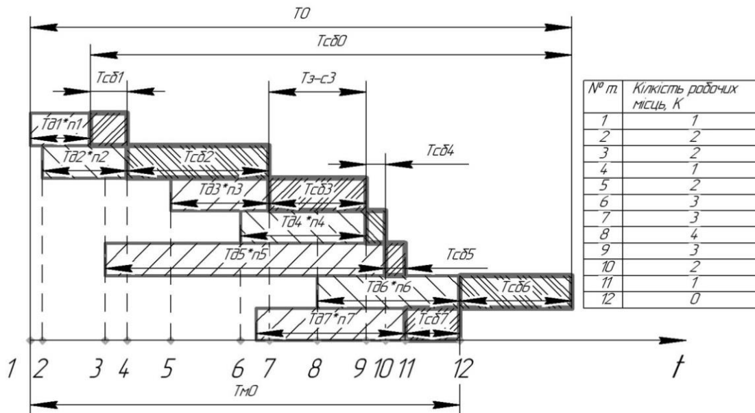
Рисунок 6.8 – Циклограма виготовлення
