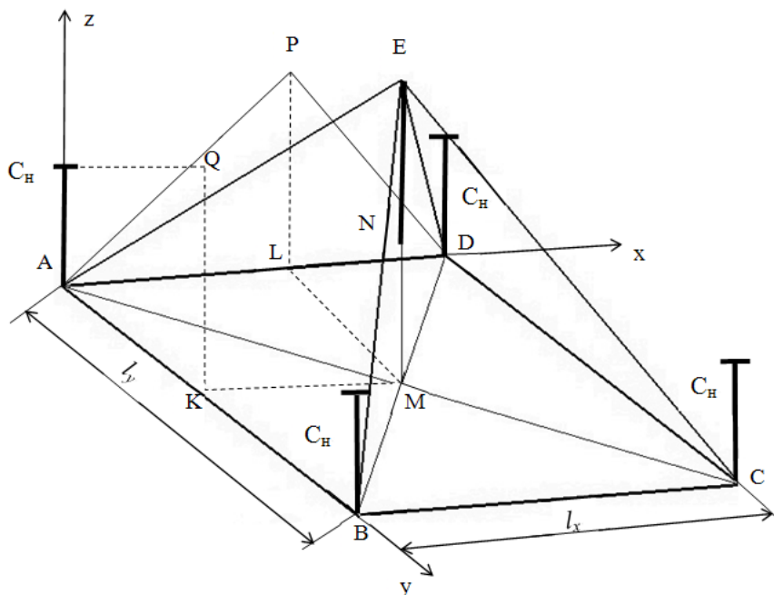
Рисунок 3.8 – Розрахункова схема октопода для визначення робочої області
