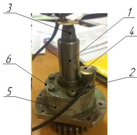
Рисунок 6.25 – Експериментальна установка
