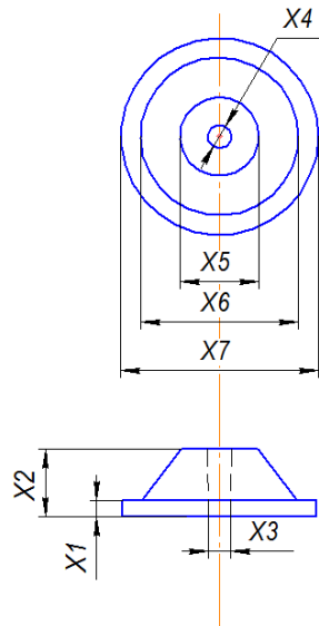
Рисунок 4.21 – Експериментальний зразок
