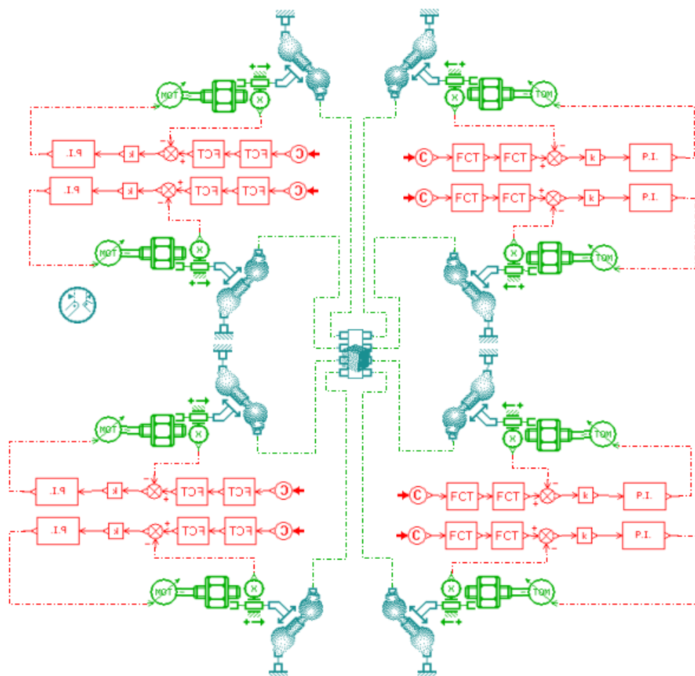
Рисунок 3.18 – Схема моделювання МПС у вигляді октопода в програмному пакеті AMESim
