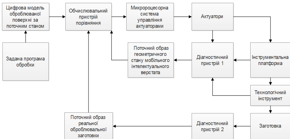
Рисунок 3.2 – Структурна схема управління мобільним верстатом із МПС
