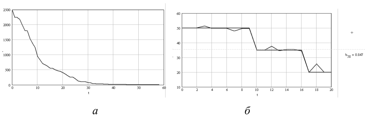
Рисунок 4.9 – Результати моделювання зношування твердосплавного різального інструменту при одночасному забезпеченні мінімуму похибки відпрацювання траєкторії (а) із дотриманням принципу найкоротшого шляху як умови мінімізації енергоємності технологічного процесу (б)
