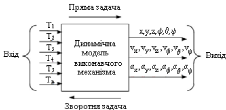
Рисунок 4.4 – Взаємозв'язок вхідних і вихідних параметрів моделі, де T_1, T_2 \dots T_n – керовані ланки МПС
