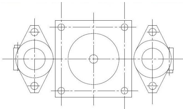
Рисунок 5.4 – Розміщення отворів для кріплення двигуна КГП і розміщення направляючих
