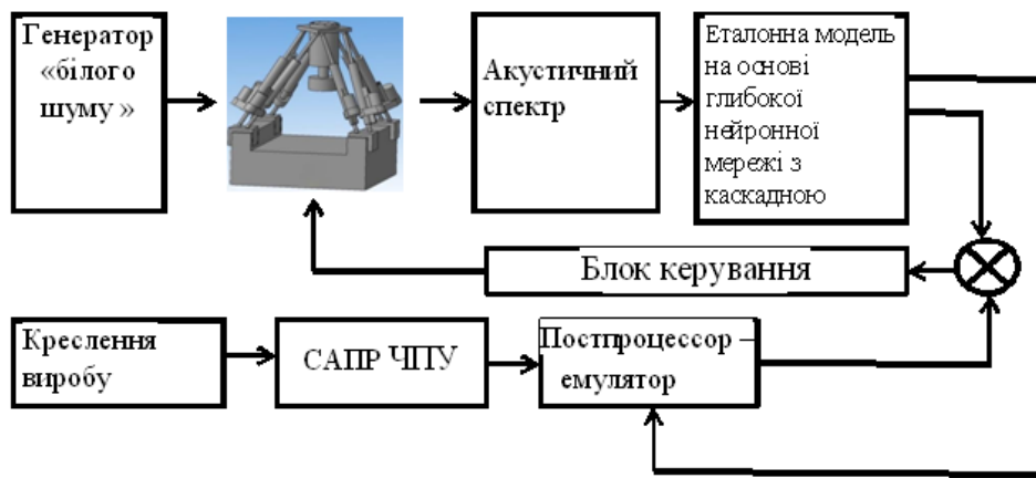
Рисунок 4.3 – Структура системи управління на глибоких нейроподібних мережах із каскадною реалізацією
