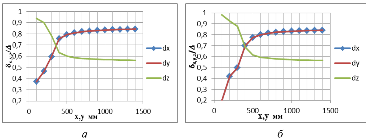
Рисунок 3.14 – Залежність похибки від довжини X при C_n : a – 300 мм; б – 500 мм
